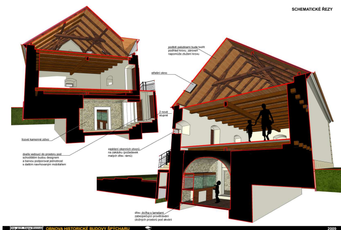
Špýchar po rekonstrukci - návrh
