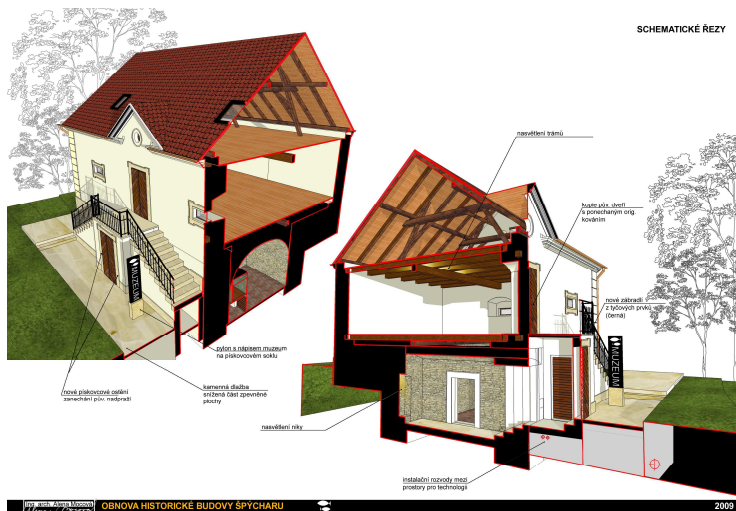
Špýchar po rekonstrukci - návrh
